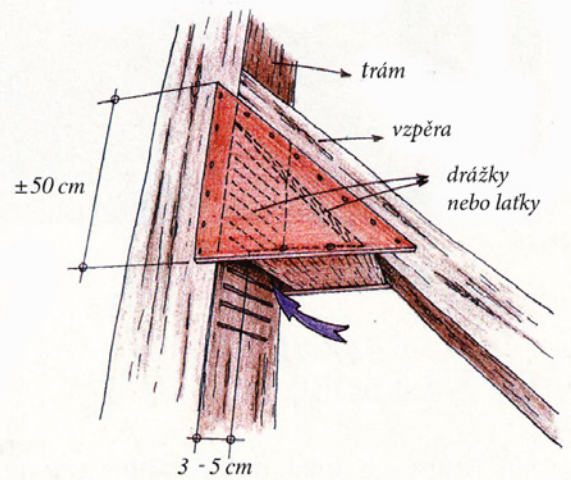
vytvoření úkrytu na rohu trámové vzpěry
