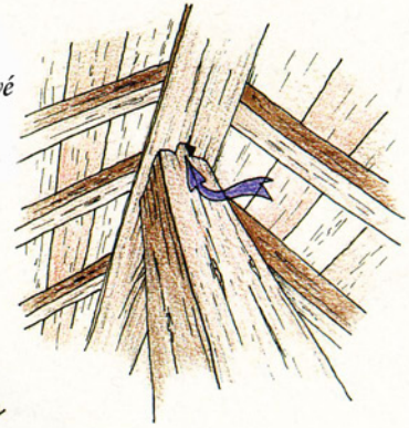
v mezeře u spoje mezi vzpěrou a krokví
