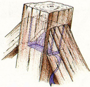
ve štěrbinách v místě napojení vzpěr do sloupku krovu
